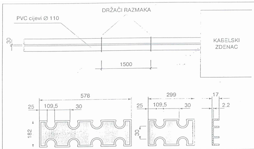
Izgled držača razmaka cijevi i način postavljanja
